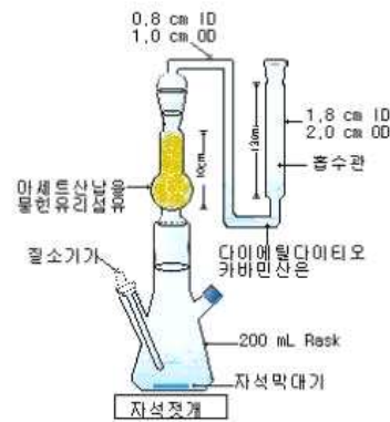
그림 1. 수소화비소 발생장치와 흡수관
