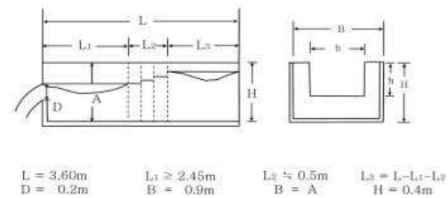
그림 8. 4각 웨어의 구조 및 치수
