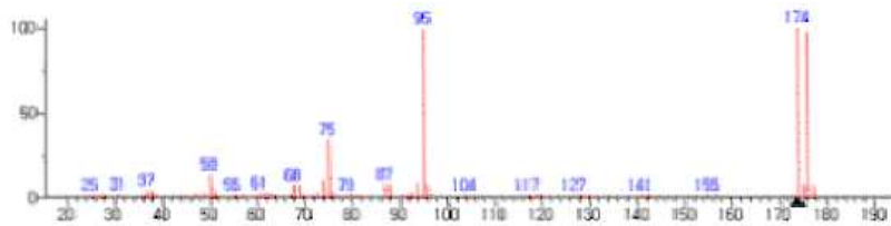
그림 4. 내부표준물질 브로모플루오로벤젠의 질량스펙트럼
