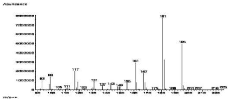
그림 3. 폼알데하이드 펜타플루오로벤질 히드라진의 질량스펙트럼
