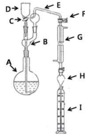
그림 1. 증류장치
