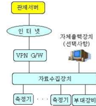
그림 1. 단일 방류구 구성도
