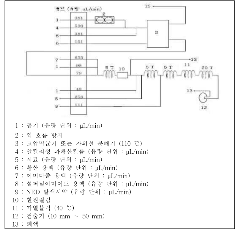
그림 1. 총 질소 분석장치의 구성도(예)
