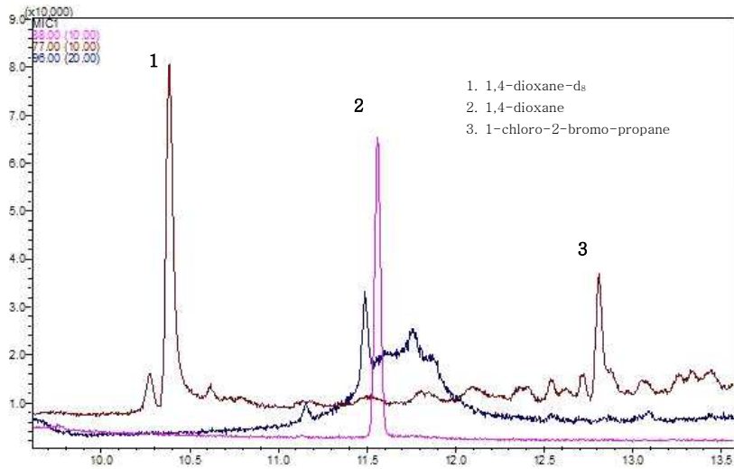
그림 1. 표준물질의 GC-MS 크로마토그램
