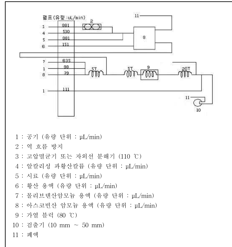
그림 1. 총인 분석장치의 구성도(예)
