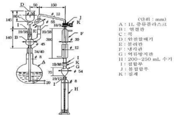
그림 1. 총 질소 증류장치
