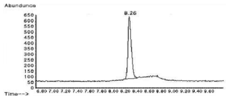
그림 1. 1,4-다이옥산의 기체크로마토그래피-질량분석기 크로마토그램 (50 \mu\text{g/L} )
