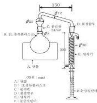
그림 1. 증류장치
