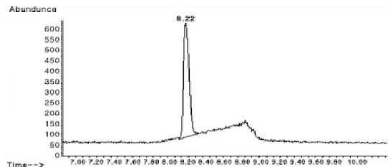
그림 2. 1,4-다이옥산-d8의 기체크로마토그래피-질량분석기 크로마토그램 (50 \mu\text{g/L} )
