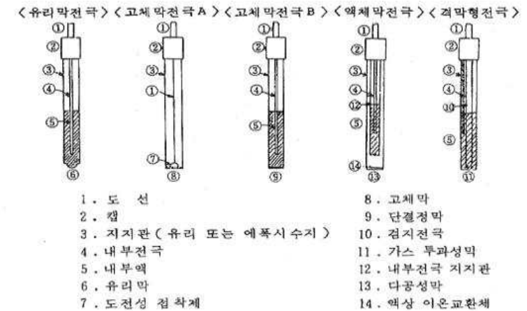
그림 1. 이온전극의 종류와 구조
