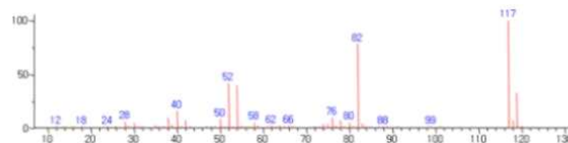
그림 4. 내부표준물질 클로로벤젠-d 5 의 질량스펙트럼
