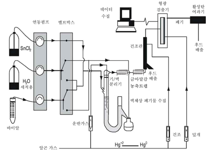
그림 1. 자동 수은 형광 분석장치
