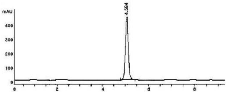
그림 1. 폼알데하이드의 고성능 액체크로마토그래피 크로마토그램 (250 μg/L)
