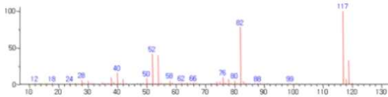
그림 4. 내부표준물질 클로로벤젠- d_6 의 질량스펙트럼
