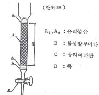
그림 1. 크로마토그래프용 알루미늄 컬럼
