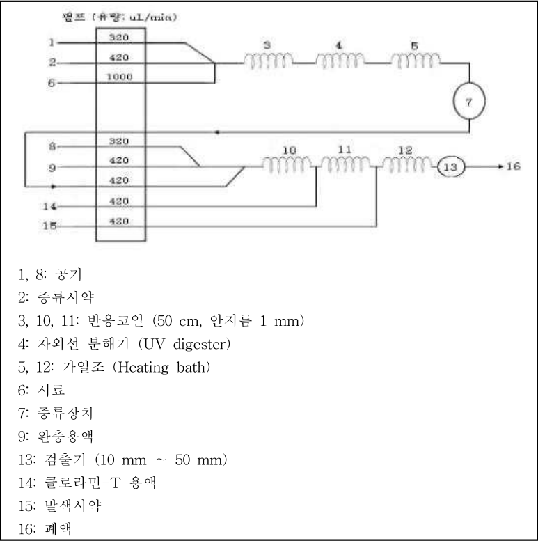
그림 1. 시안 분석장치의 구성도(예)
