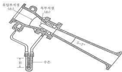
그림 1. 벤튜리미터
