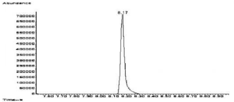
그림 1. 폼알데하이드 펜타플루오로벤질 히드라진의 기체크로마토그래피-질량분석기 크로마토그램 (250 \mu g/L)
