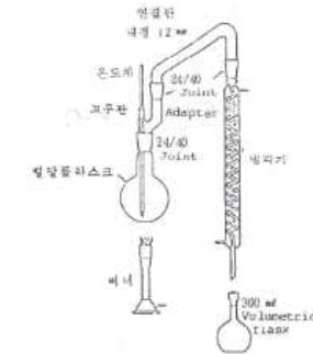
그림 1. 직접 증류장치
