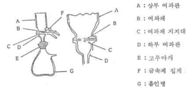
그림 1. 여과장치
