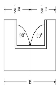
그림 6. 4각웨어의 절단
