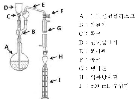
그림 1. 증류장치
