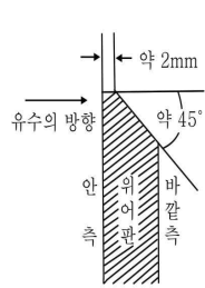
그림 3. 웨어판의 가장자리
