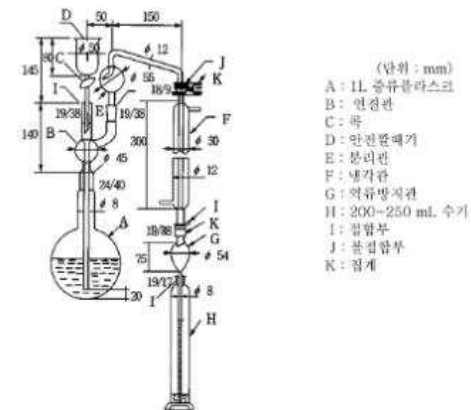
그림 1. 시안증류장치 구성도
