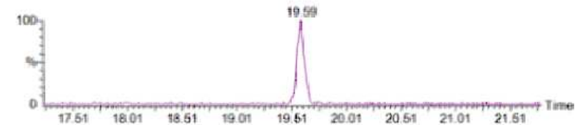
그림 3. 내부표준물질 브로모플루오로벤젠의 크로마토그램
