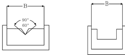
그림 1. 웨어의 구조
