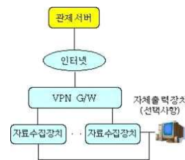
그림 2. 복수 방류구 구성도(1)
