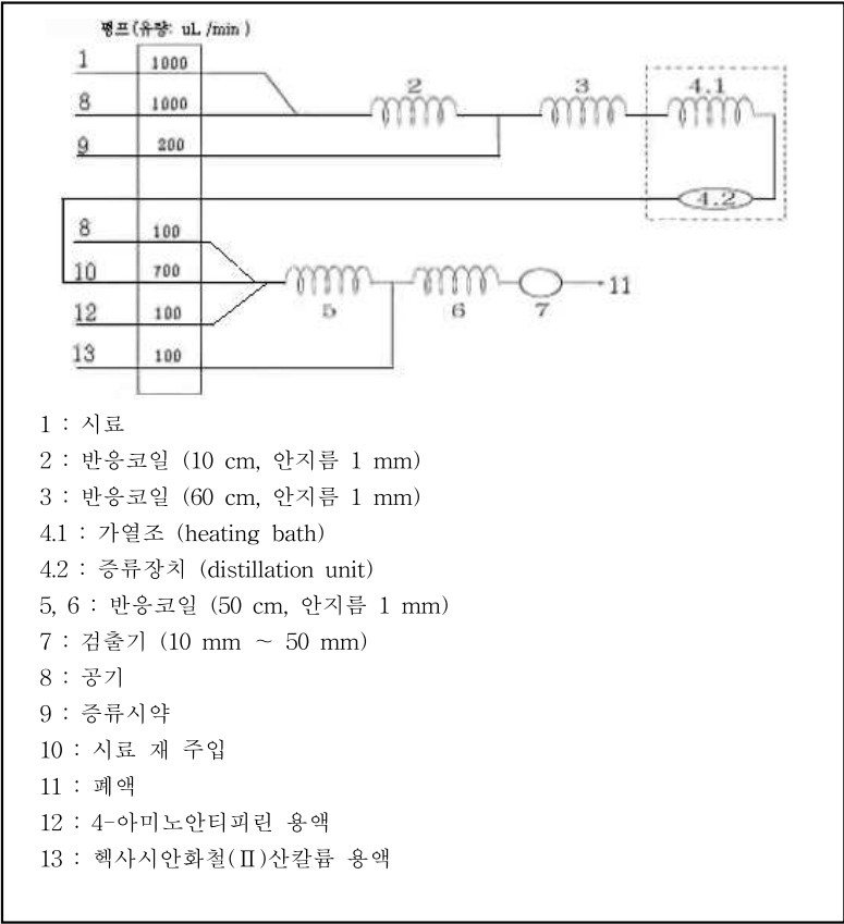
그림 1. 페놀류 분석장치의 구성도(예)
