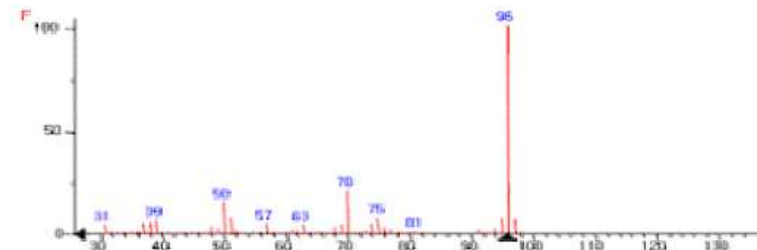
그림 4. 플루오로벤젠의 질량스펙트럼
