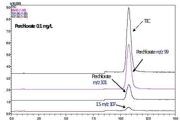
그림 2. 퍼클로레이트 표준물질의 LC-MS 크로마토그램
