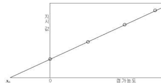
그림 2. 표준물첨가법에 의한 검정곡선
