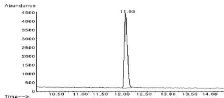
그림 2. 1,4-다이옥산-d8의 크로마토그램 (50 µg/L)
