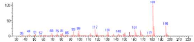
그림 2. 유도체화된 폼알데하이드의 질량스펙트럼
