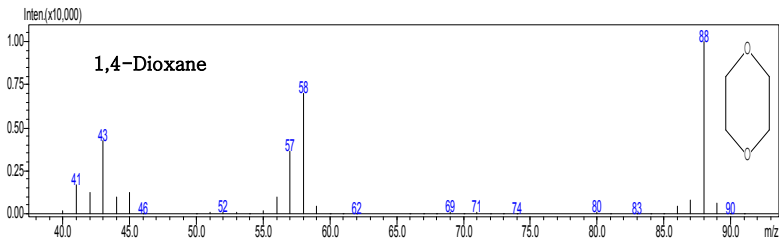
그림 2. 1,4-다이옥산의 질량스펙트럼
