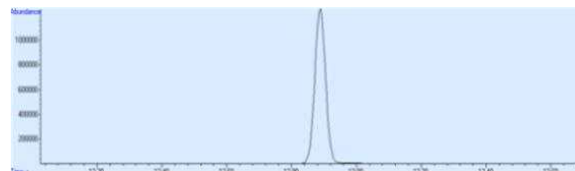
그림 3. 내부표준물질 클로로벤젠-d 5 의 크로마토그램
