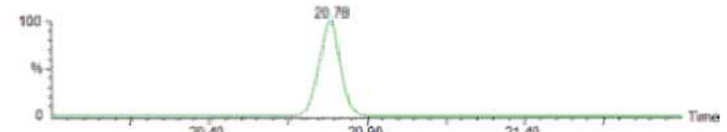
그림 1. 유도체화된 폼알데하이드의 크로마토그램
