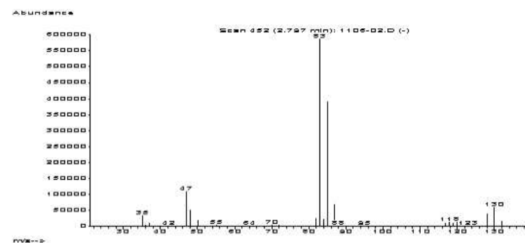
그림 2. 휘발성유기화합물의 질량스펙트럼
