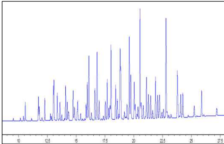
그림 5. PCBs(Aroclor-1242:1248:1254:1260) 크로마토그램(예)
