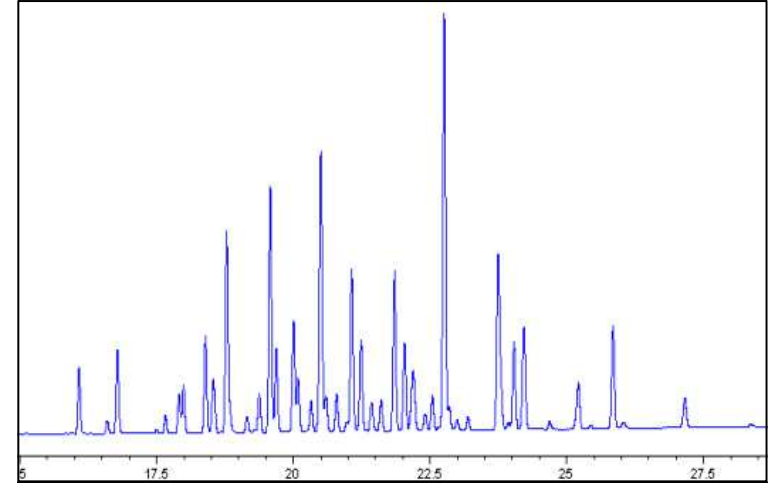
그림 4. PCBs(Aroclor-1260) 크로마토그램(예)
