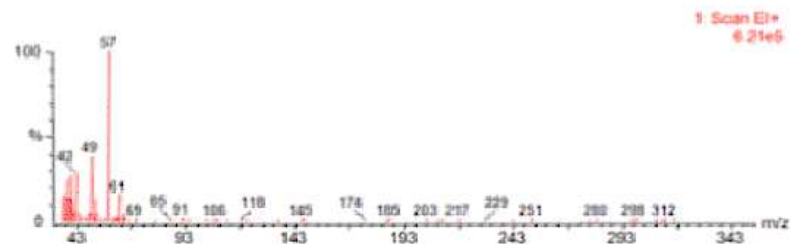
그림 2. 에피클로로하이드린의 질량스펙트럼
