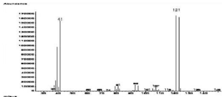
그림 4. 1,2-디브로모피로판의 질량스펙트럼
