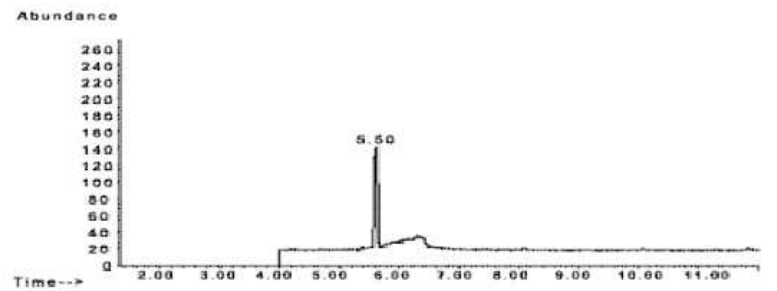
그림 2. 1,4-다이옥산-d8의 기체크로마토그래피-질량분석기 크로마토그램 (5 μg/L)
