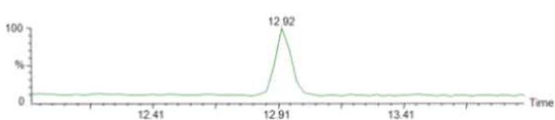
그림 3. 내부표준물질 클로로벤젠- d_5 의 크로마토그램
