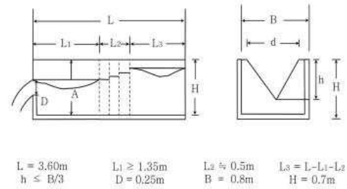
그림 7. 직각 3각 웨어의 구조 및 치수
