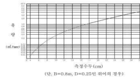
그림 11. 직각 3각 웨어의 수두와 유량
