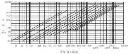
그림 15. 수위, 유량 환산그래프
