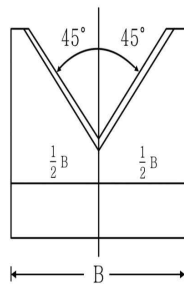
그림 5. 직각 3각웨어의 절단
