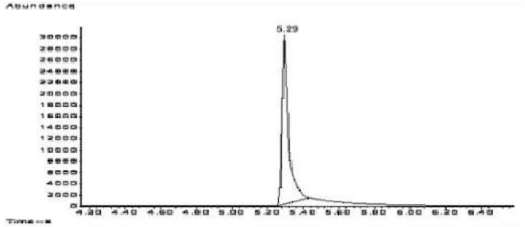
그림 2. 1,2-디브로모피로판의 기체크로마토그래피-질량분석기 크로마토그램 (50 \mu g/L)
