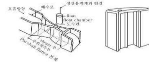
그림 13. 파살수로의 개략도
