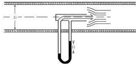
그림 4. 피토우 (Pitot) 관
