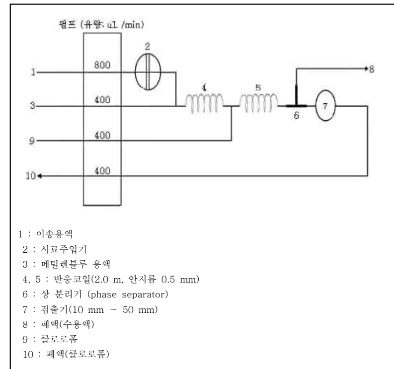
그림 1. 음이온 계면활성제 분석장치의 구성도(예)
