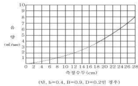
그림 12. 4각 웨어의 수두와 유량
