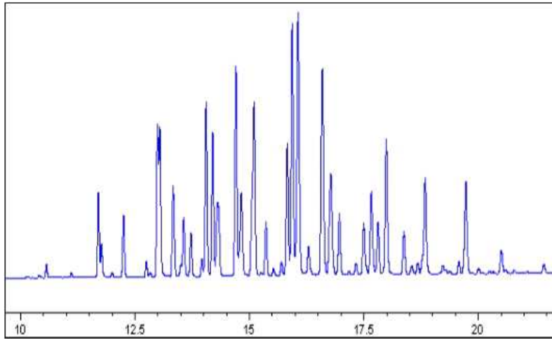
그림 2. PCBs(Aroclor-1248) 크로마토그램(예)
