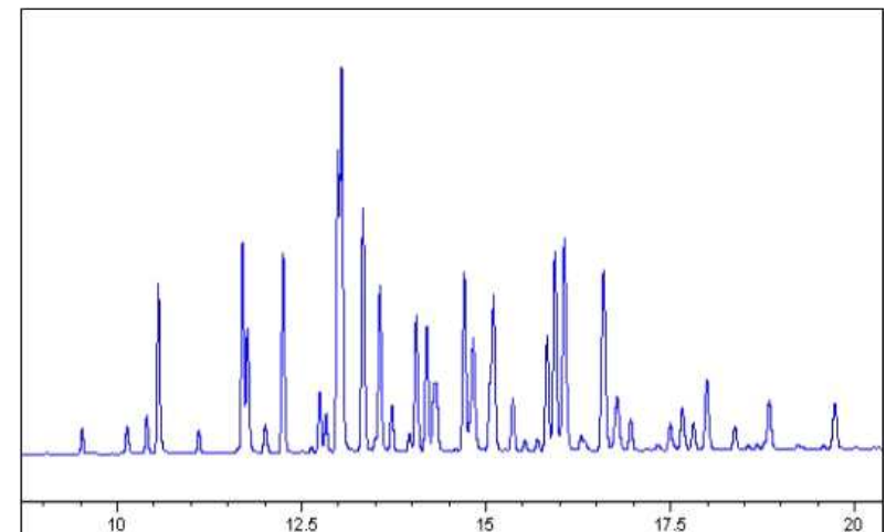
그림 1. PCBs(Aroclor-1242) 크로마토그램(예)
