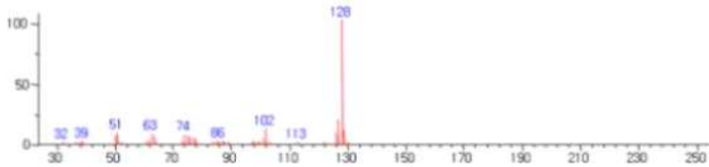
그림 2. 나프탈렌의 질량스펙트럼
