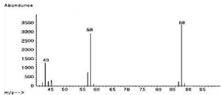
그림 3. 1,4-다이옥산의 질량스펙트럼
