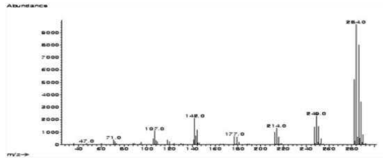
그림 2. 헥사클로로벤젠의 질량 스펙트럼
