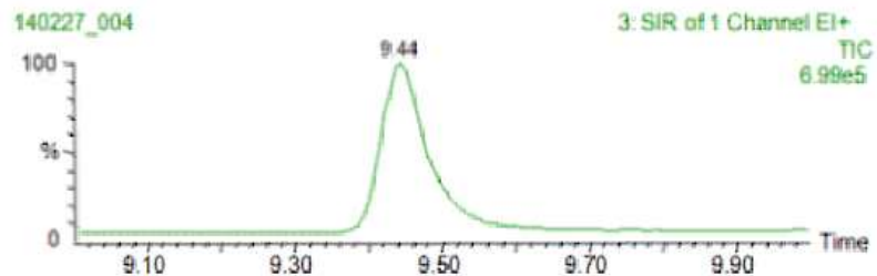
그림 3. 플루오로벤젠의 크로마토그램
