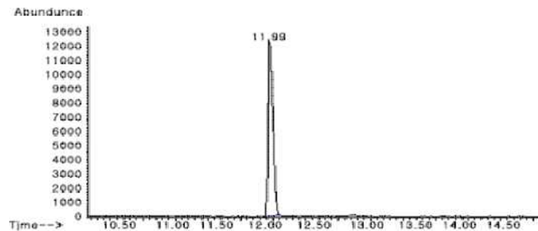
그림 1. 1,4-다이옥산의 크로마토그램 (100 µg/L)
