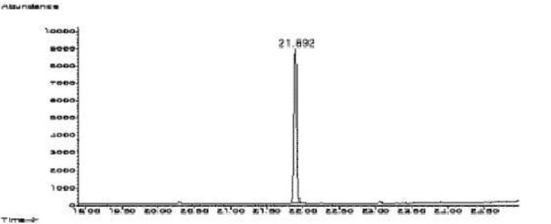
그림 1. 헥사클로로벤젠의 기체크로마토그래피-질량분석기 크로마토그램 (0.02 µg/L)
