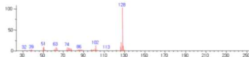
그림 2. 나프탈렌의 질량스펙트럼
