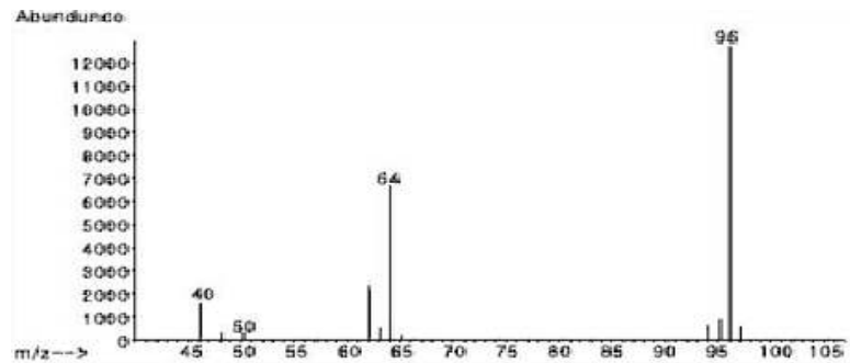
그림 4. 1,4-다이옥산-d8의 질량스펙트럼
