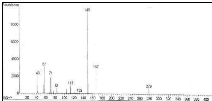
그림 1. 디에틸헥실프탈레이트의 질량스펙트럼(예)
