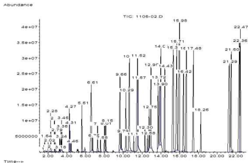
그림 1. 휘발성유기화합물 표준물질의 GC-MS 크로마토그램(예)
