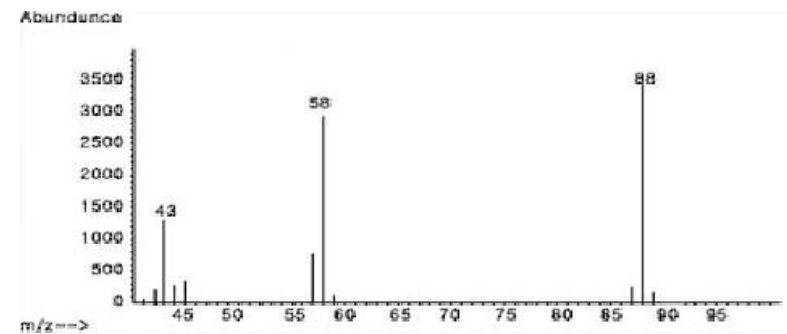
그림 3. 1,4-다이옥산의 질량스펙트럼
