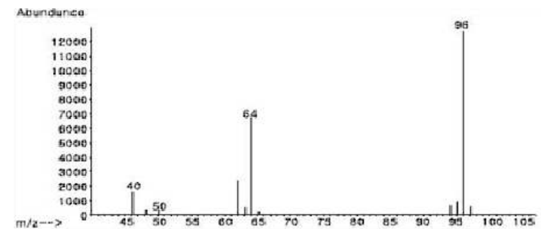
그림 4. 1,4-다이옥산-d8의 질량스펙트럼
