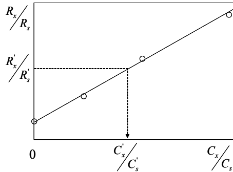
그림 3. 내부표준법에 의한 검정곡선
