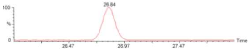
그림 1. 나프탈렌의 크로마토그램
