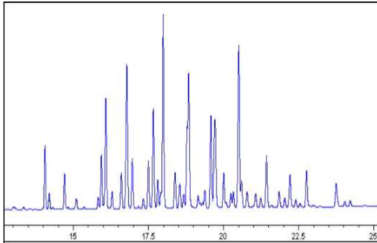
그림 2. PCBs(Aroclor-1248) 크로마토그램(예)
