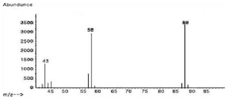
그림 3. 1,4-다이옥산의 질량스펙트럼
