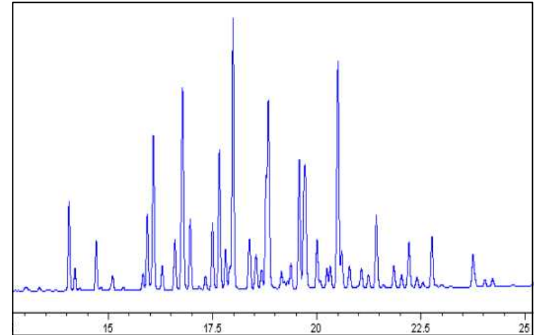
그림 3. PCBs(Aroclor-1254) 크로마토그램(예)
