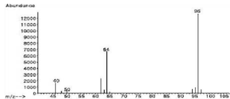
그림 4. 1,4-다이옥산-d8의 질량스펙트럼
