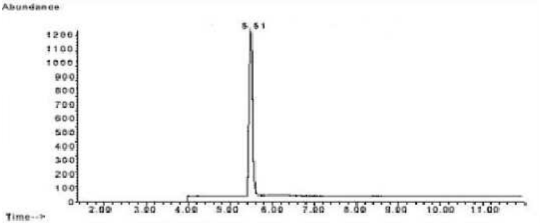
그림 1. 1,4-다이옥산의 기체크로마토그래피-질량분석기 크로마토그램 (50 μg/L)
