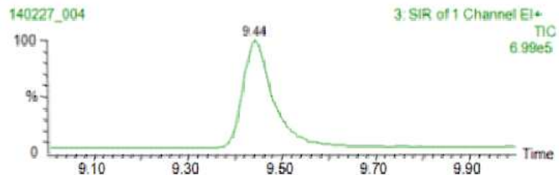
그림 1. 에피클로로하이드린의 크로마토그램
