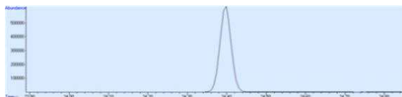
그림 1. 나프탈렌의 크로마토그램
