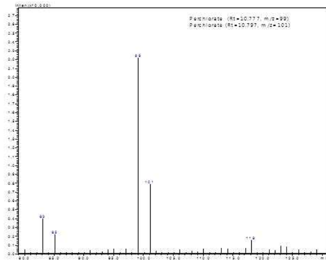
그림 3. 퍼클로레이트의 질량스펙트럼
