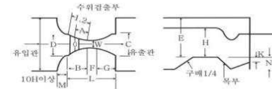
그림 14. 파살수로의 구조 및 유형
