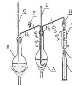
그림 2. 수증기 증류장치
